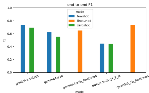
Slika 4.2. End-to-end F1 grafik po modelu/režimu
